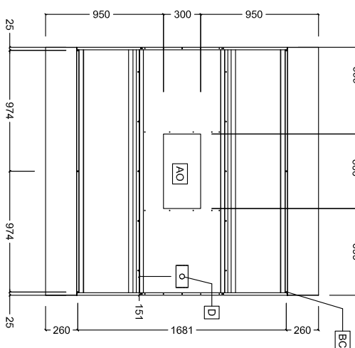
Felülnézet
